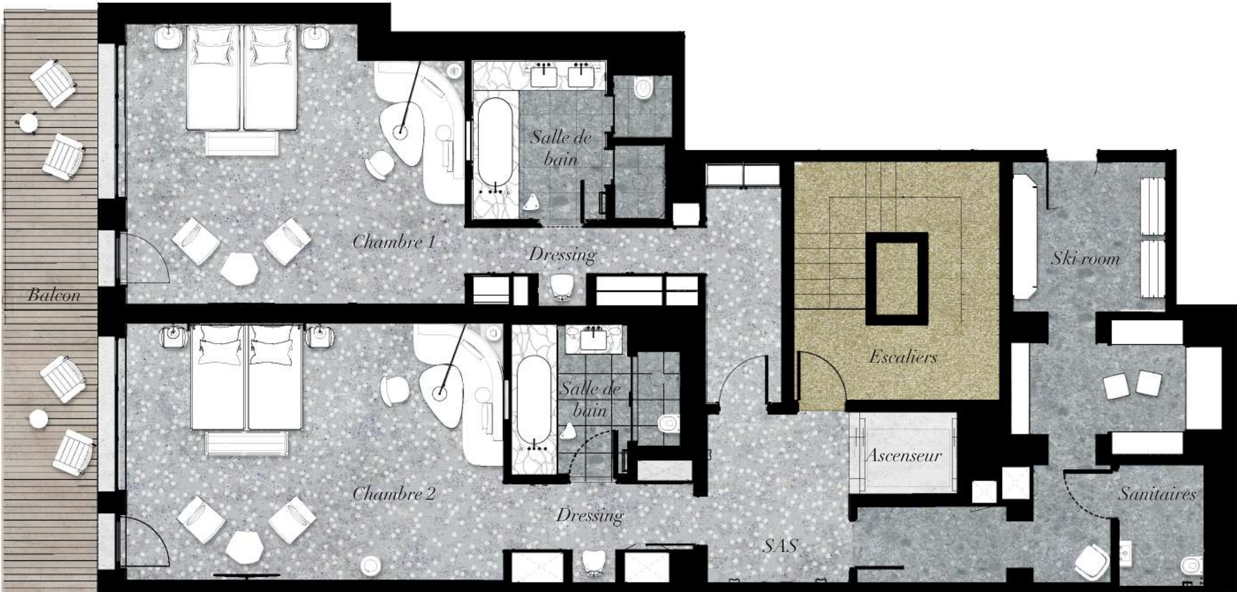
CHALET ELEONORE Etage 0
